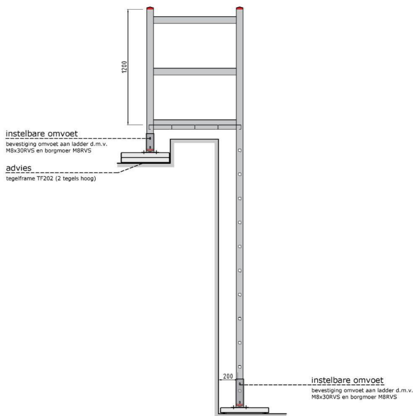
Doorsnede gevelladder type GLC-3
