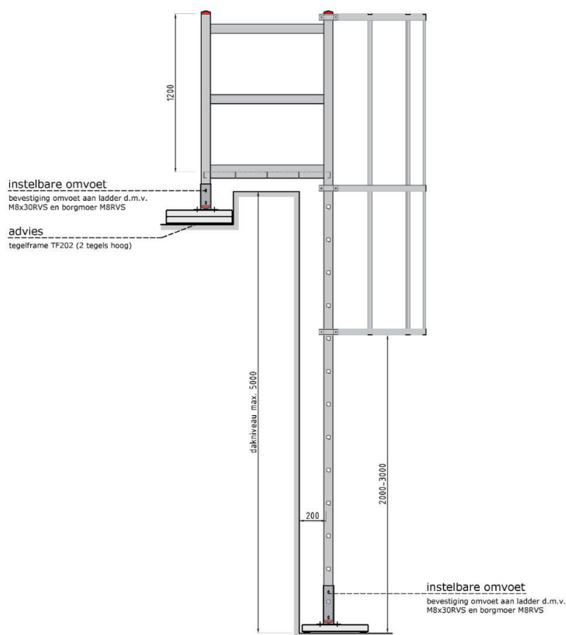
Doorsnede kooiladder type KLC-3
