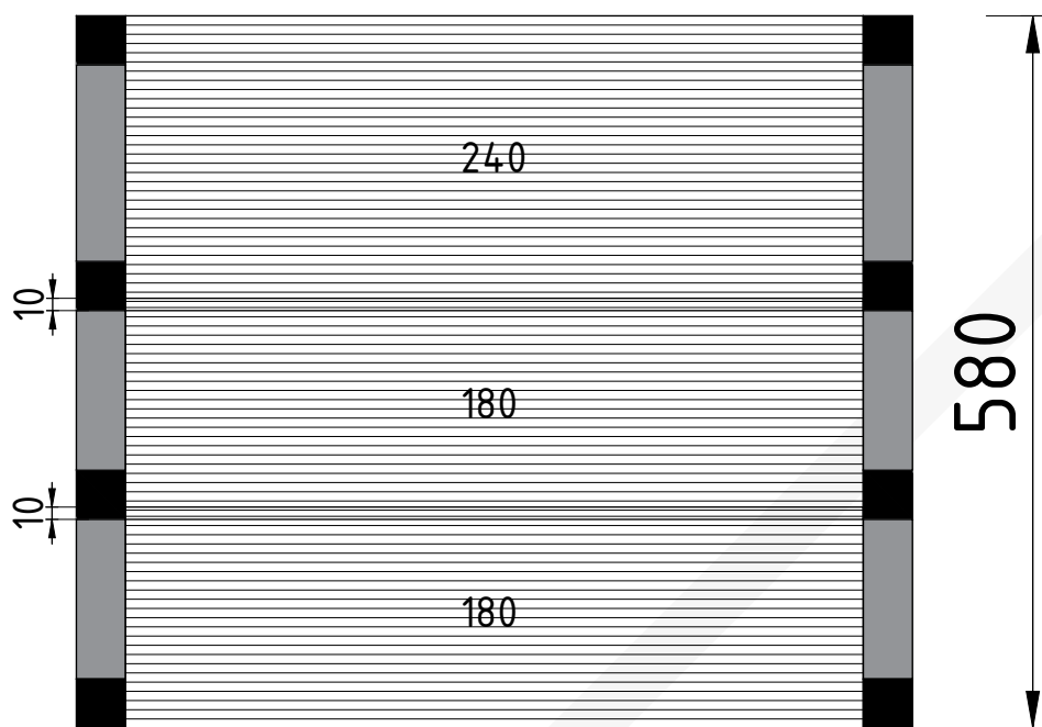
bovenaanzicht
