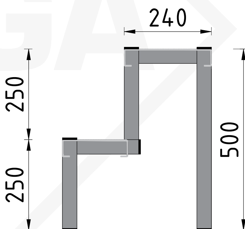
doorsnede
