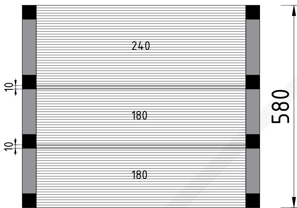
bovenaanzicht
